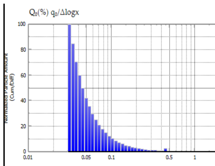
Gambar 4. Hasil penentuan sebaran ukuran larutan supernatan isolat BES 6A yang mengandung koloid nanopartikel zink oksida dengan konsentrasi precursor \text{ZnSO}_4 0.2 g/ml menggunakan PSA
