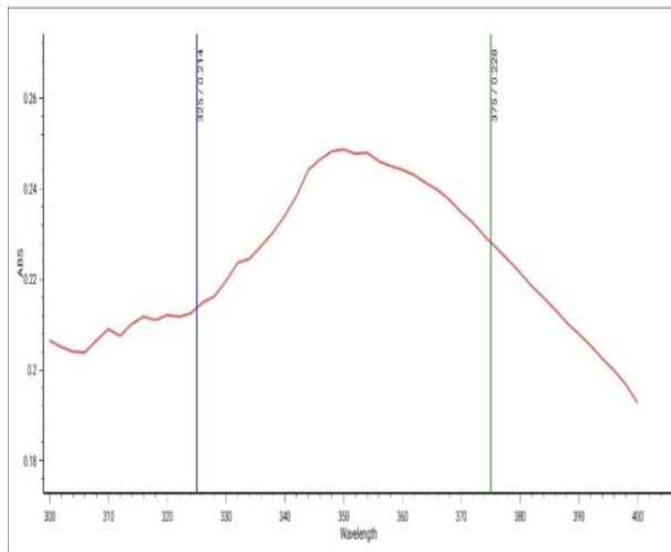
Gambar 2. Hasil penentuan serapan maksimum larutan supernatan isolat bioreduktor BES 6A yang mengandung koloid nanopartikel zink oksida dengan konsentrasi precursor \text{ZnSO}_4 0.2 g/ml menggunakan spektrofotometer UV-Vis
