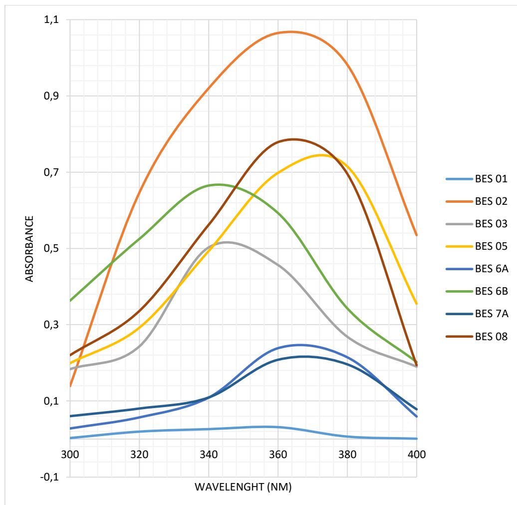
Gambar 2. Profil hasil penentuan panjang gelombang maksimal dari supernatan isolat bioreduktor BES 01, BES 02, BES 03, BES 05, BES 6A, BES 6B, BES 7A, dan BES 08 yang mengandung nanopartikel zink oksida pada hari ke tujuh sintesis dimana x: panjang gelombang (nm) dan y: nilai absorbansi.
