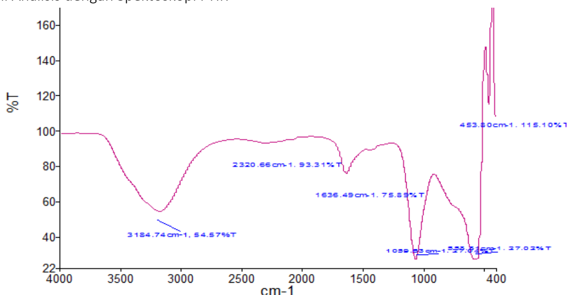
Gambar 3. Hasil penentuan gugus fungsi rendemen nanopartikel zink oksida yang disintesis menggunakan isolat bioreduktor BES 6A dengan konsentrasi precursor ZnSO 4 0.2 g/ml menggunakan FTIR
